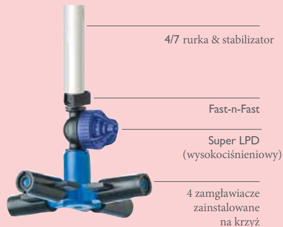
PRZEPŁYW ZAMGŁAWIACZA KRZYŻOWEGO (l/h)
