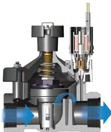
Przekrój zaworu PESB
