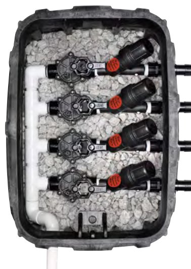
Cztery zestawy sterowania sekcją w standardowej skrzynce zaworowej
