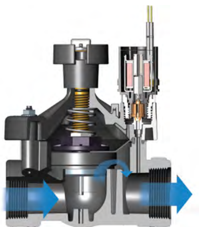
Przekrój zaworu PEB
