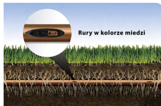
Podziemna linia kroplująca XFS z technologią ekranu miedzianego (Copper Shield™)
