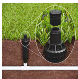
Dysza SQ na zraszacz 1800 Zespół korpusu
